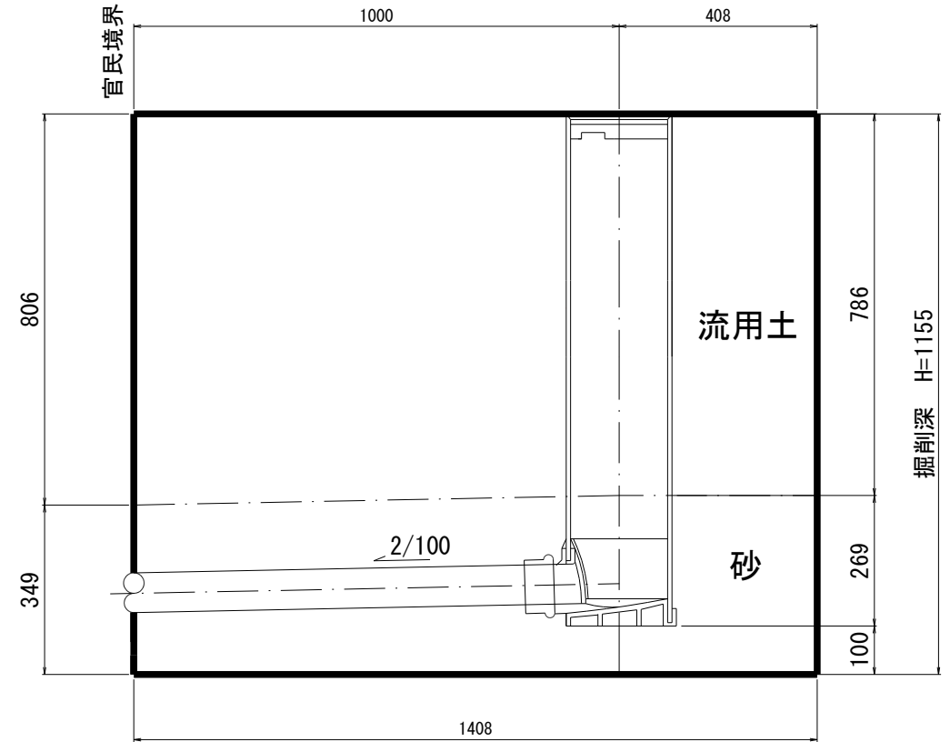
公共汚水柵：フリーインパートタイプ H=1000
